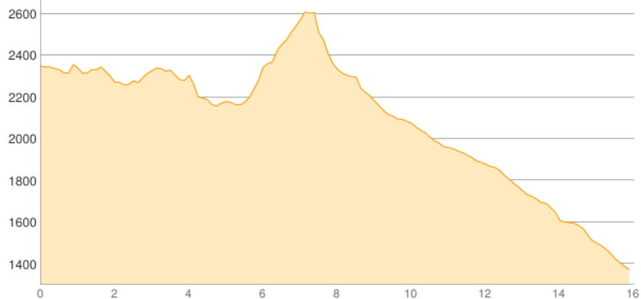
Höhenprofil
