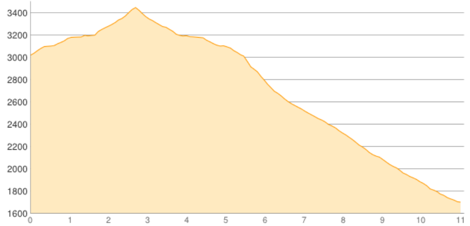
Höhenprofil
